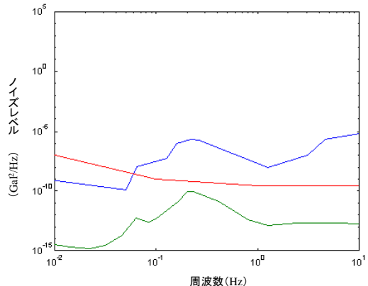
エピセンサのノイズモデル(2g, ローノイズ)
